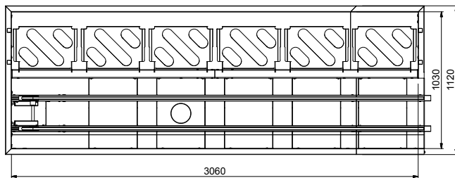
Boven aanzicht
